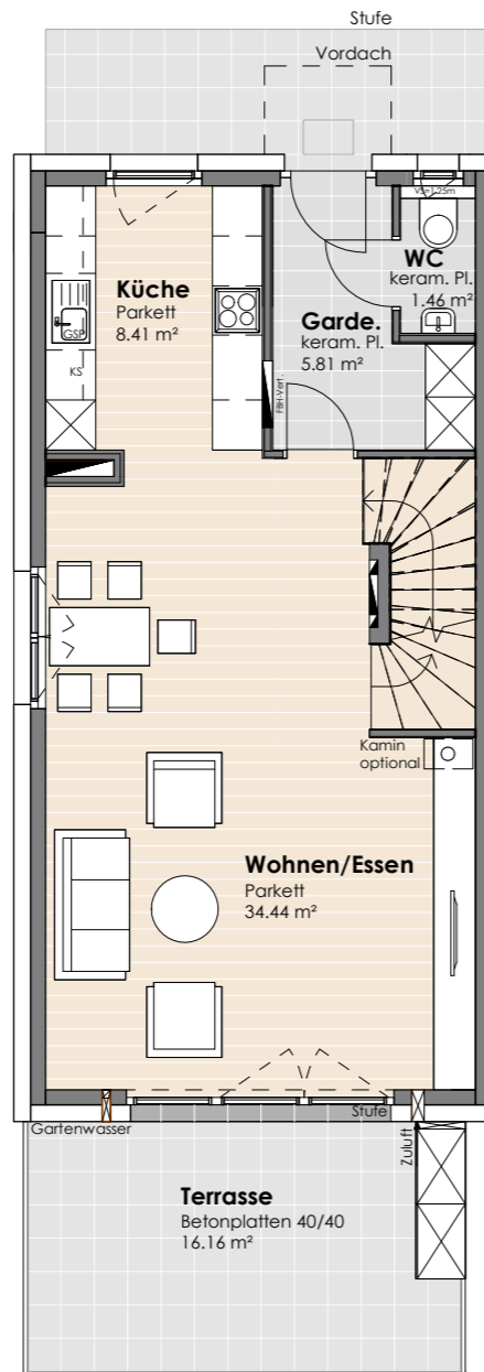
ERDGESCHOSS
