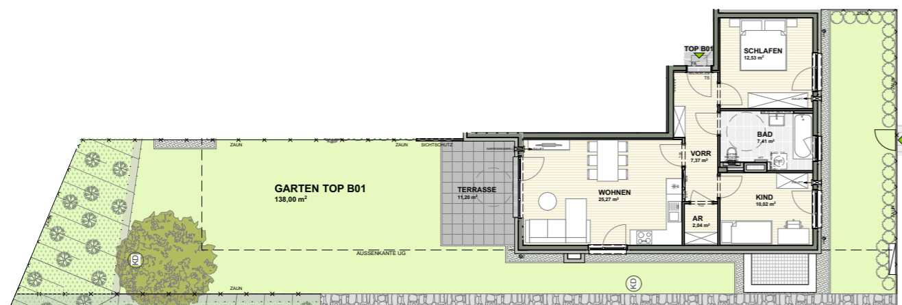
ÜBERSICHTSPLAN 1:200
