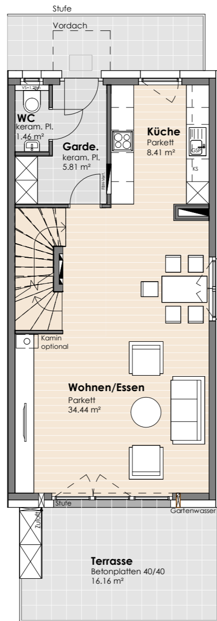
ERDGESCHOSS
