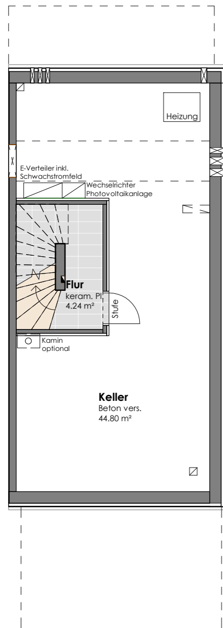
KELLERGESCHOSS
