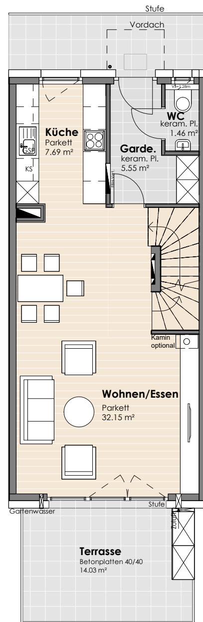
ERDGESCHOSS
