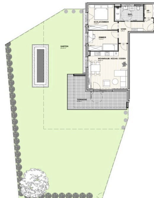
Übersichtsplan 1:200
