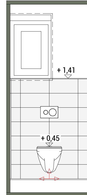
Ansicht 4
