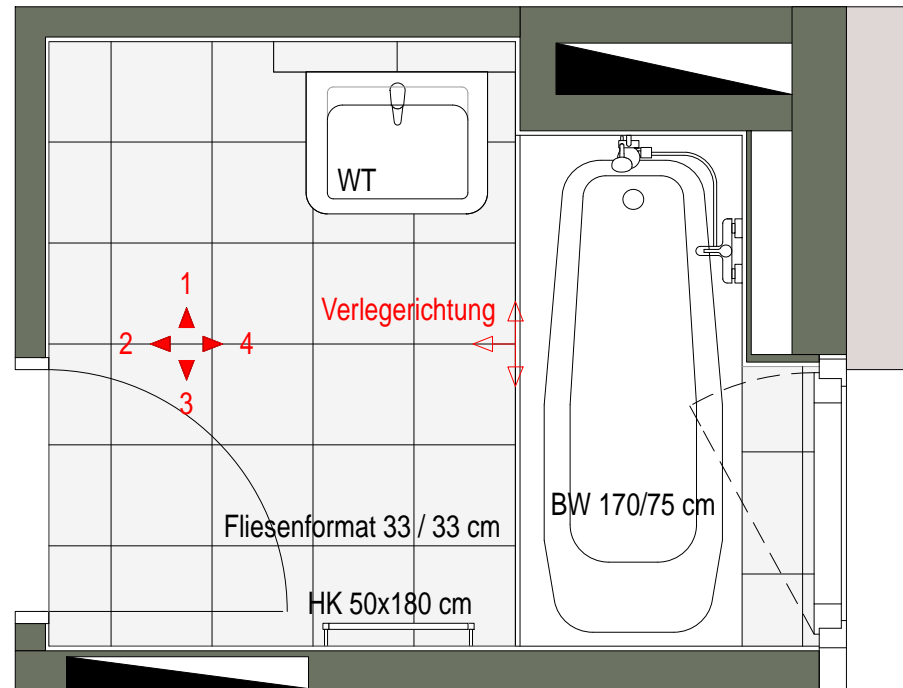
Grundriss
