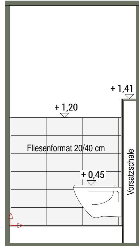
Ansicht 1
