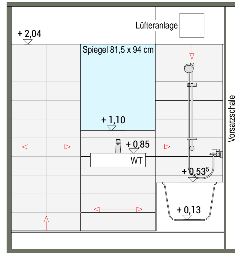
Ansicht 4
