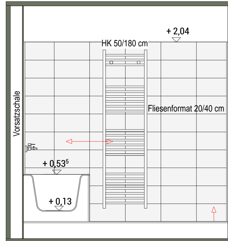
Ansicht 3
