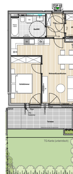
Übersichtsplan 1:200
